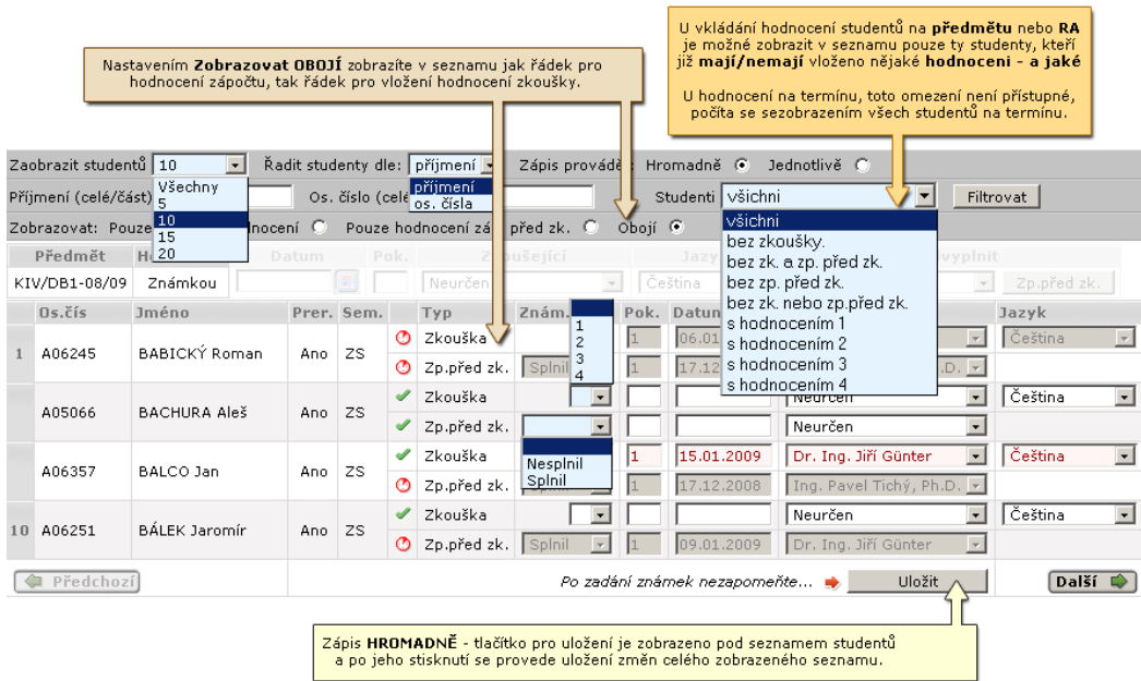
Obrázek 3.16: Popis omezujícího filtru formuláře pro vkládání hodnocení – první část.
