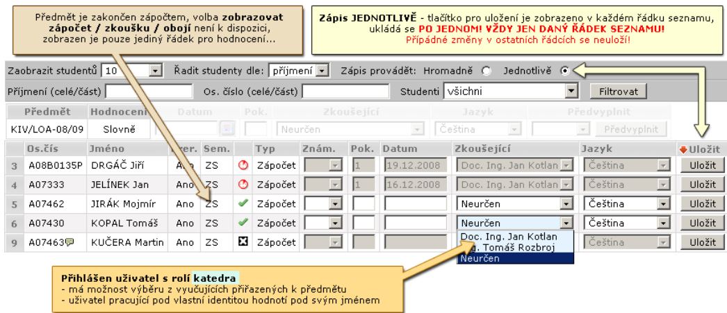
Obrázek 3.17: Popis omezujícího filtru formuláře pro vkládání hodnocení – druhá část.
