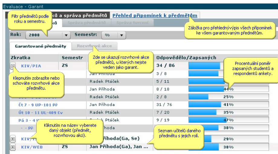
Obrázek 3.104: Výběr akademického roku a seznam garantovaných předmětů.
